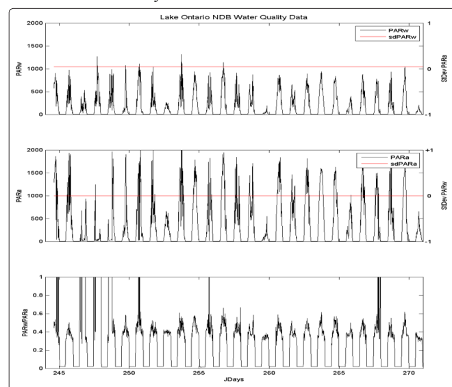
Figure 4: PAR sensor data
